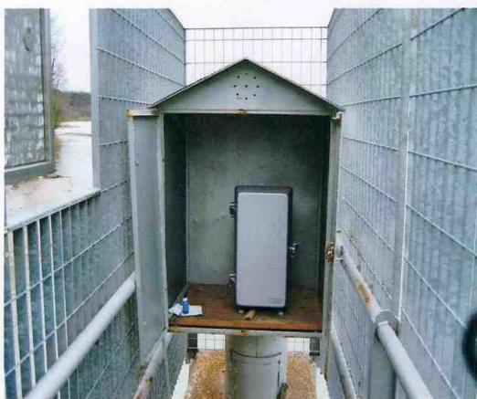
IDROMETROGRAFO SIAP INSTALLATO IN CABINA
