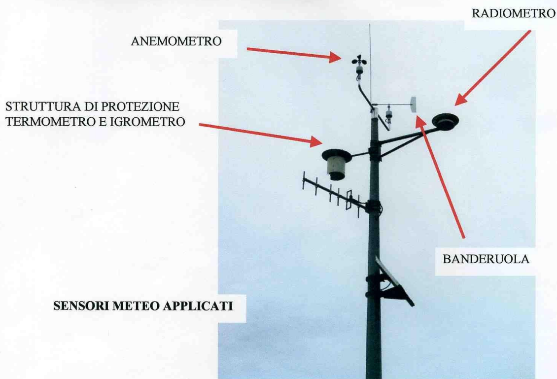
Figura 137 - strumenti elettronici installati nella stazione della Protezione Civile ad Arba
