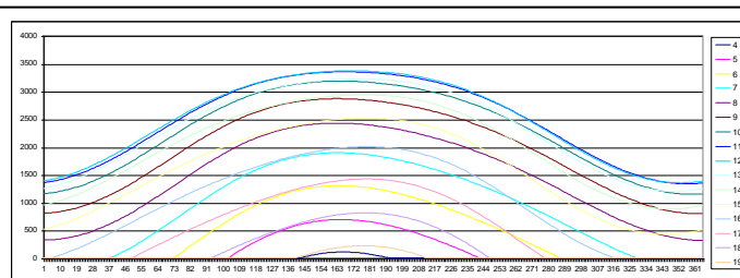
Figura 18 - Andamento della Radiazione Solare oraria (ore UTC) teorica a livello del suolo in assenza di nubi per una latitudine pari a 46°N e longitudine di 13.5°E [kJ/ m 2 ora]
