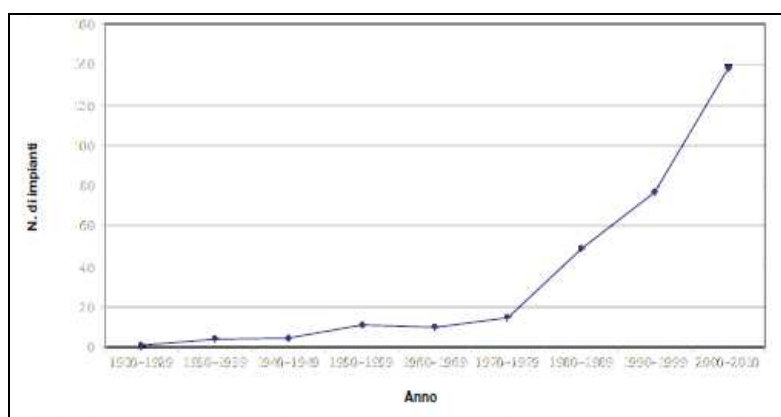
Figura 92- Incremento degli impianti idroelettrici. Fonte: elaborazione RAFVG, servizio Idraulica.
