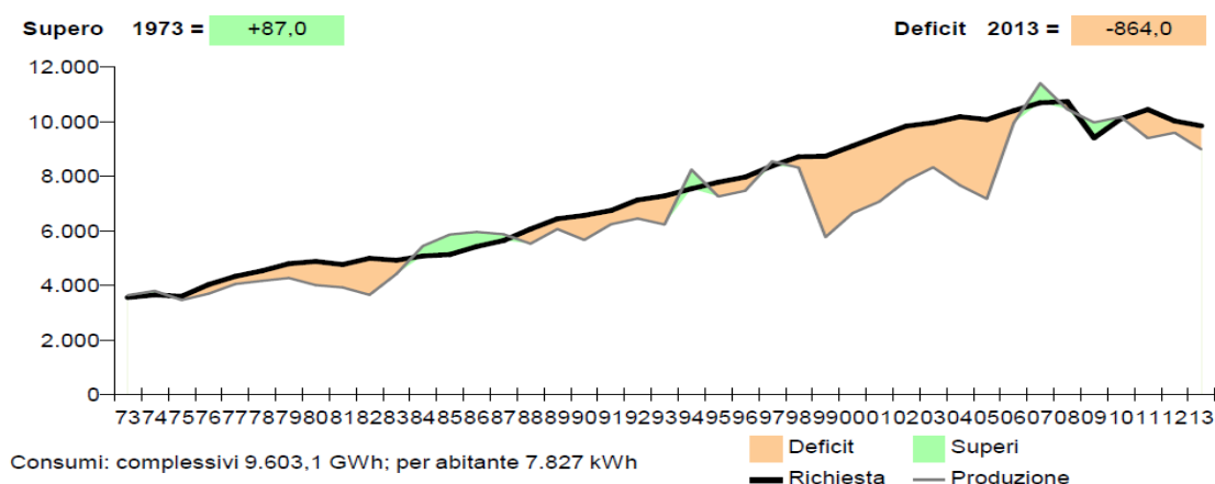
Figura 95 - Produzione di energia elettrica regionale. Fonte: TERNA, "Dati statistici sull'energia elettrica in Italia", 2013.
