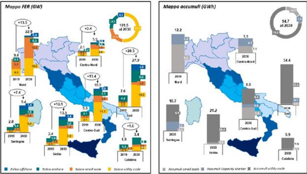
Figura 7.17. Dettaglio evoluzione capacità FER (GW) e capacità totale accumuli (GWh) al 2030 nello scenario FF55 126 .
