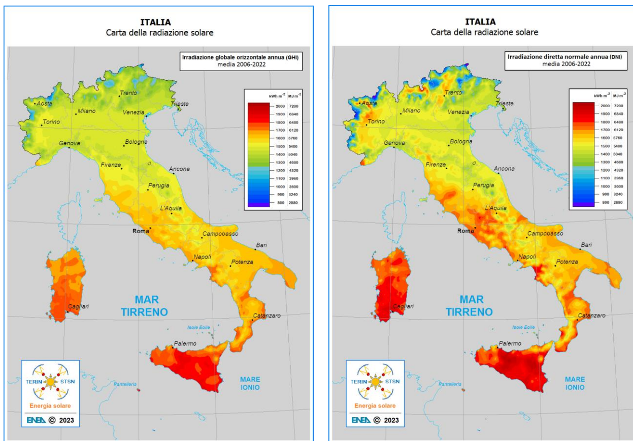
Figura 7.2. Mappa radiazione solare media 2006-2022, GHI a sinistra, e DNI a destra. Fonte ENEC.
