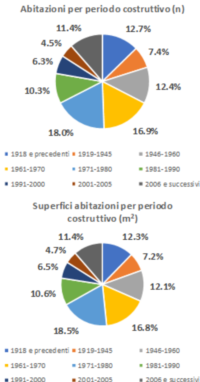
Figura 4.56. Percentuale delle abitazioni (sopra) e delle superfici delle abitazioni (sotto) per epoca di costruzione (Fonte: Elaborazioni ENEA su dati ISTAT).
