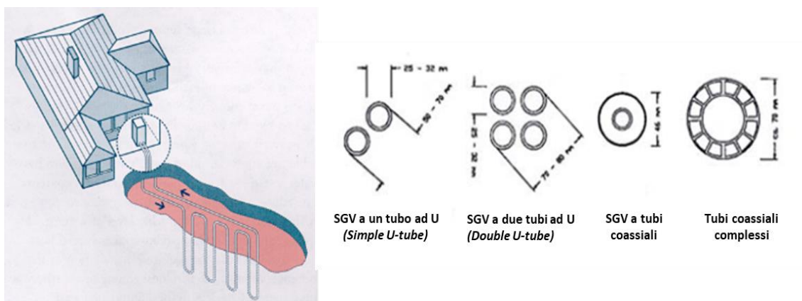
Figura 4.18. Sonde geotermiche di tipo verticale e schema rappresentativo di diverse configurazioni.
