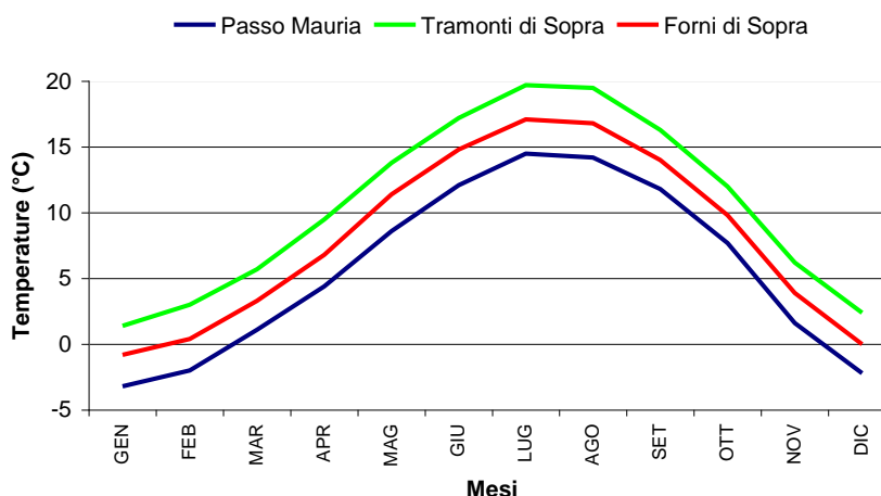
Figura IV. 1 – Andamento delle temperature medie mensili registrate a Passo Mauria, Tramonti di Sopra e Forni di Sopra, anni 1961-1990. (Fonte dei dati: ARPA FVG).
